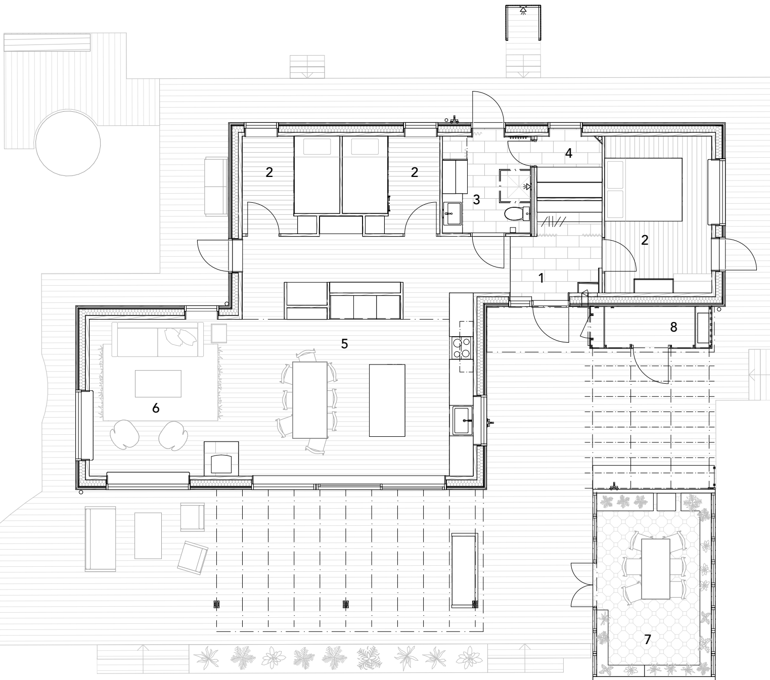
ENTRÉPLAN
