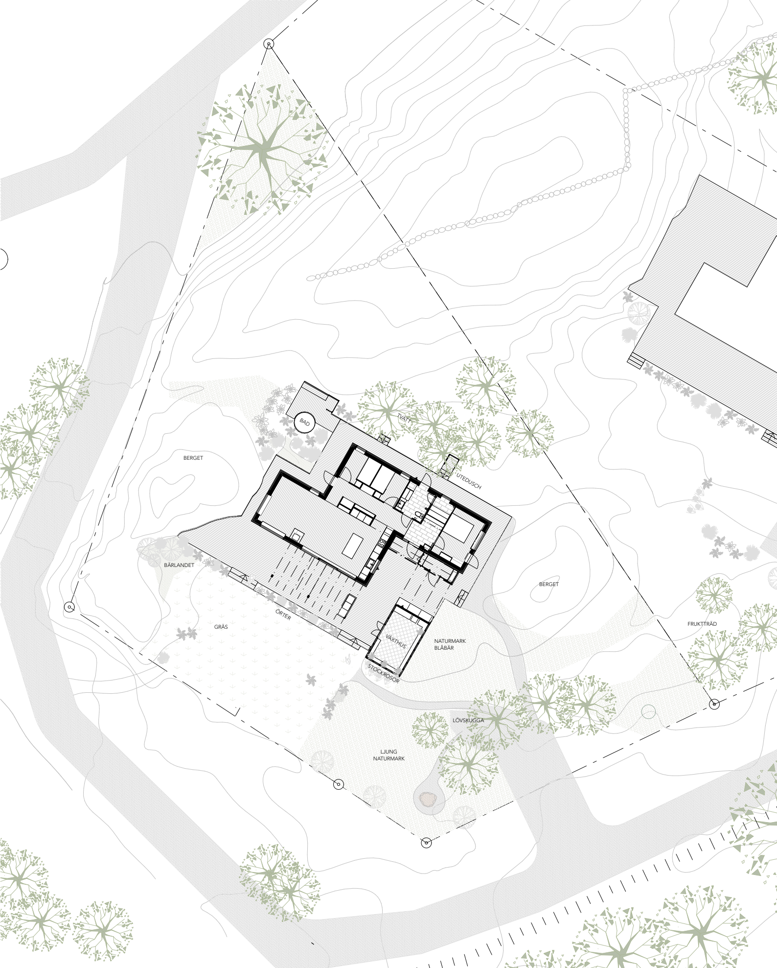
VILLA SIV, SITUATIONSPLAN SKALA 1:300
