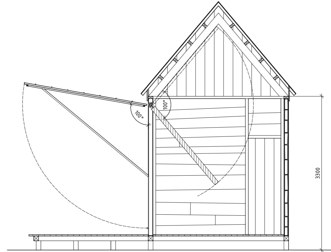
SEKTION AA
